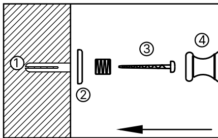
ART. 99100-CR
