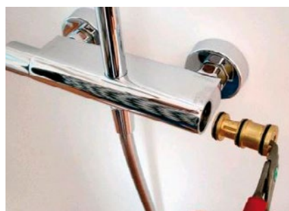
3. Inserire l'adattatore
